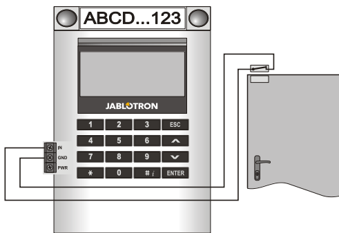
Obr. 4: Pripojenie detektora otvorenia dverí
