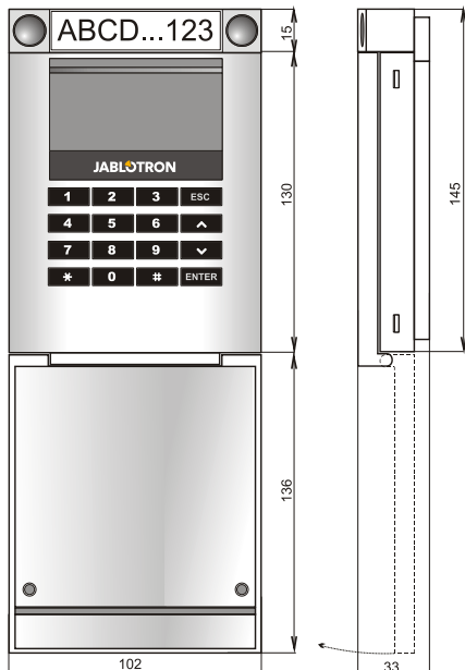
Obr. 5: Rozmery modulu
