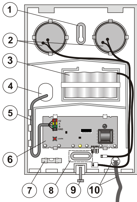
Obr. 1: 1 – montážny otvor; 2 – elektroakustické meniče; 3 – NiCd akumulátor; 4 – otvor pre privedenie káblu; 5 – kábel zbernice; 6 – elektronika sirény; 7 – integrovaná libela; 8 – otvor pre montáž sirény na stenu s detekciou sabotáže; 9 – skrutka krytu sirény; 10 – lanko so sponou istiace vrchný kryt (stlačením západky ho možno ľahko odpojiť)
